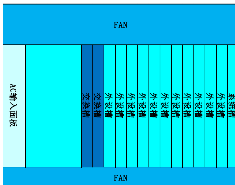
后视图
