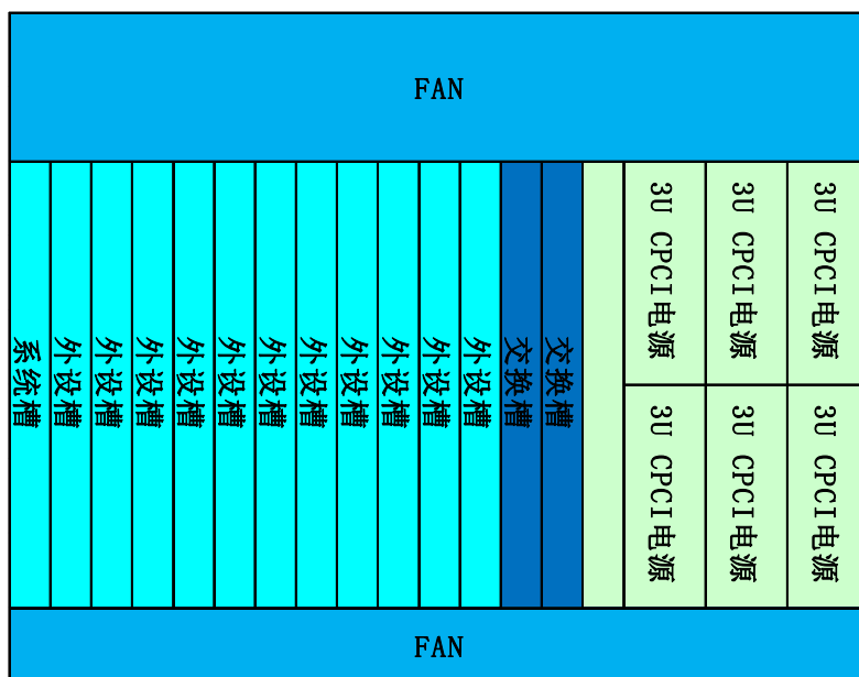
前视图
